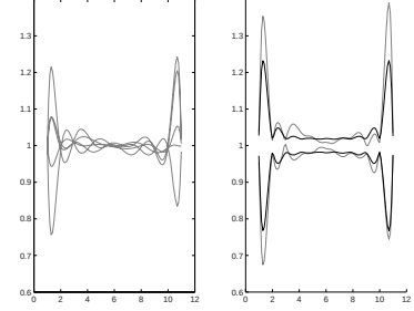
Fig. 4. Lagrange DSA 5 samples+CSA
