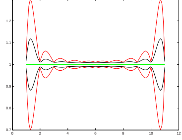
Fig. 2. Lagrange, Interval+CSA
