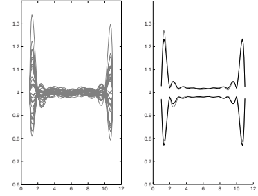
Fig. 6. Lagrange DSA 30 samples+CSA
